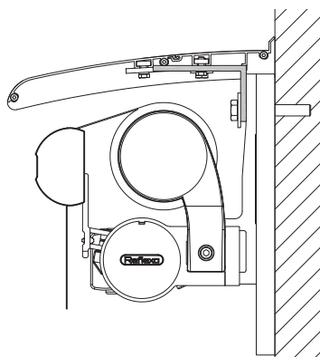
Montage an Wandkonsole mit Konsolplatte
