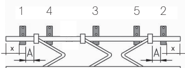
Anlage mit 3 Armen und 3 bzw. 5 Konsolen
