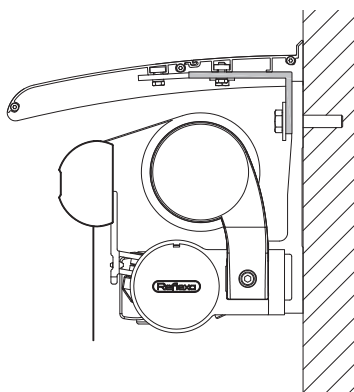
Montage an Wandkonsole
