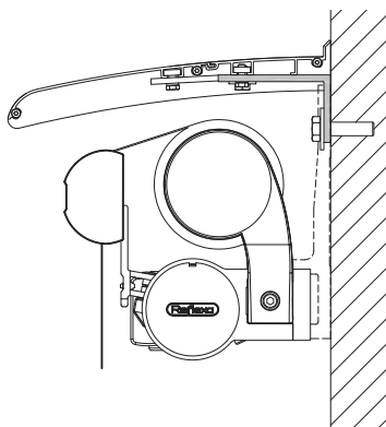
Montage direkt an die Wand
