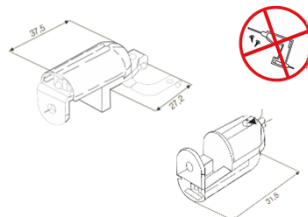
Optional: Jalousie Klemmträger
