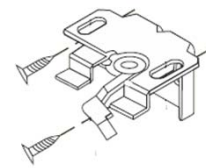
2. Jalousiehalter als Wandmontage anschrauben
